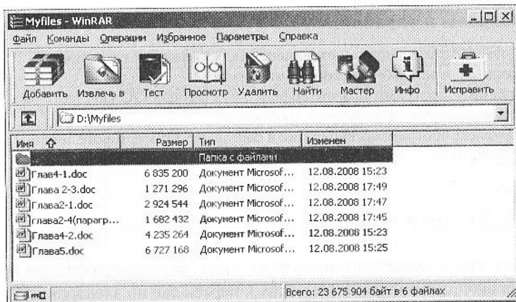
Рис. 3.22. Интерфейс WinRAR
