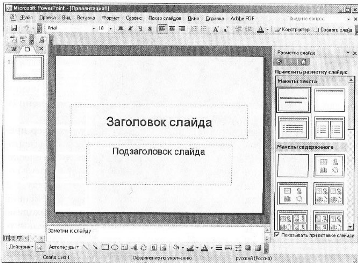
Рис. 4.32. Разметка слайда
