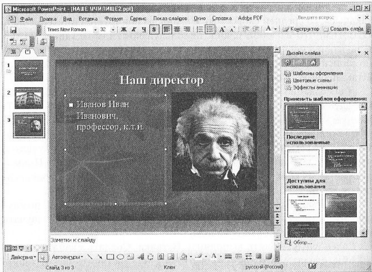
Рис. 4.36. Слайд 3
