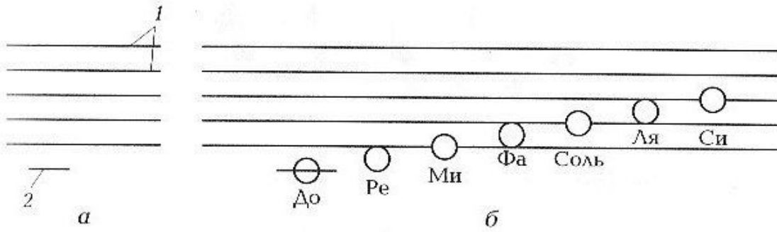
Рис. 2.12. Нотная запись:
