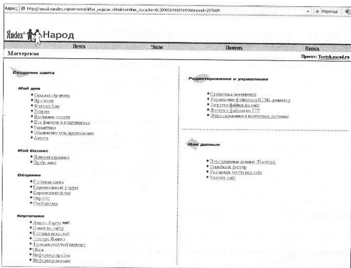
Рис. 6.11. Окно «Мастерская»
